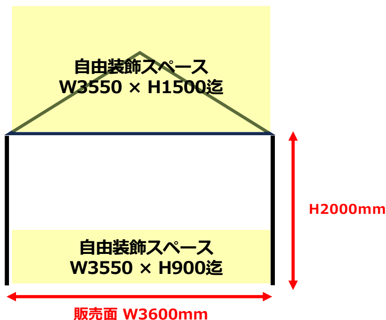
【立面図】
